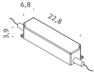
185W / LIN ALI 36
