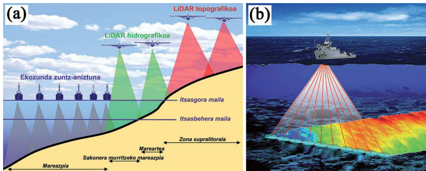
1. irudia. Erabili diren sentsoreen lan egiteko era aurkeztzen duten modelo kontzeptualak: (a) hiru teknika ezberdinen sakonera-ahalmena; (b) sorta anitzeko ekozundak itsas hondoko datuak jasotzen dituen era. ARG.: CONTINENTAL SHELF PROJECT ©.
