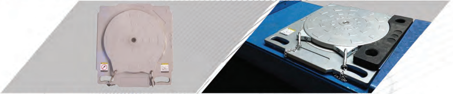
ALUMINIUM TURNABLE PLATES, 2 PCS. Obrotnice aluminiowe 2szt. / Alu-Drehteller, 2 Stk. / Алюминиевые поворотные плиты, 2 шт. VIS-AK011 Dimensions / Wymiary / Abmessungen / Размеры - 510 x 470 x 50 mm
