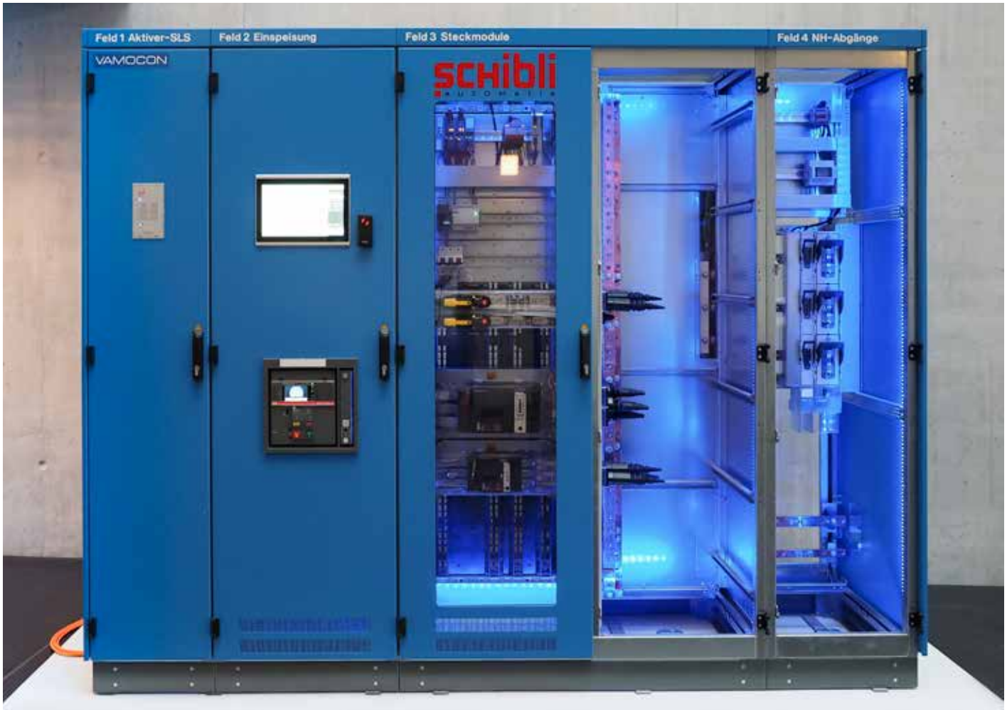
Die Vamocon-Muster-Schaltschrankanlage beinhaltet auch einen aktiven Störlichtbogen und kann für Messen oder Events zu Demozwecken genutzt werden.
