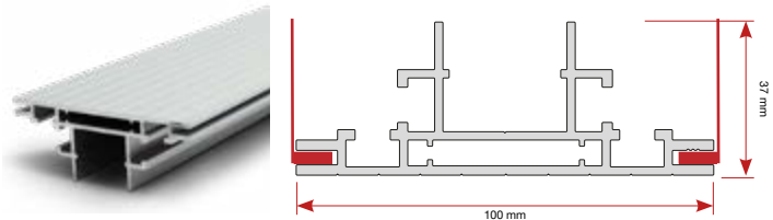
Dubbsidig profil, fristående, 100 mm IS-9665
