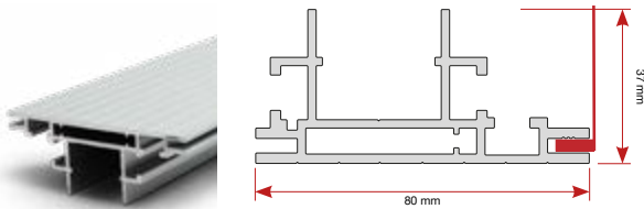
Enkelsidig profil, väggmontage, 80 mm IS-9647
