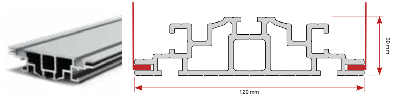
Dubbsidig profil, inbyggd, 120 mm IS-9332
