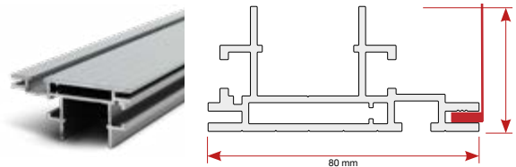
Enkelsidig profil, inbyggd, 80 mm IS-9664
