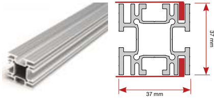
SYSTEM-RAM PROFIL Profillängd (3100 mm) IS-9097
