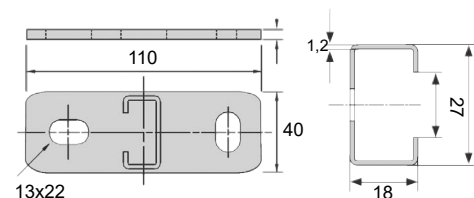
Détail platine de fixation
