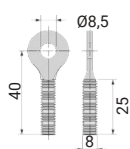
SLES M8x25 Anneau de suspension
