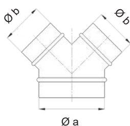
Schéma YV
