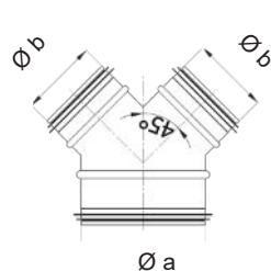
Schéma YVJ
