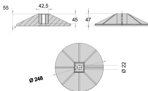
Dimensions BASE-FOOT
