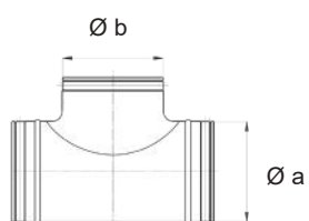
Schéma TCPJ
