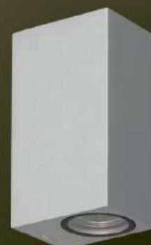
K1301G. Aluminio. 2×GU10. 16×7×7,5cm. Gris. IP54.
