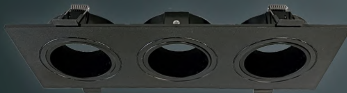
P2300N. Policarbonato. 3×GU10. 252×92mm. Orientable. Negro.
