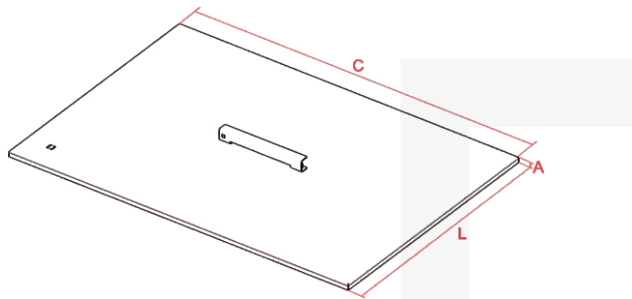
Figura 6 – Dimensões.
