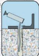
Pastroni vrimën dhe fryni pluhurin me ajër
