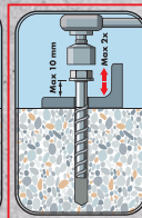
Shtrengoni bulonën e ankerimit me një çift rotullues
