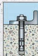
Shtërëngoni bulonën e ankerimit me një çift rotullues
