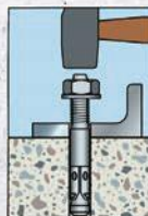
Instaloni ankerin me kujdes në vrimën e hapur
