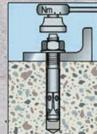
Shtrengoni bulonën e ankerimit me një çift rotullues
