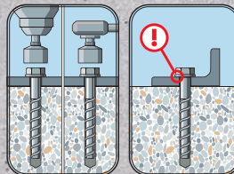
Instaloni ankerin me kujdes në vrimën e hapur
