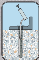
Pastroni vrimën dhe fryni pluhurin me ajër
