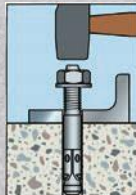
Instaloni ankerin me kujdes në vrimën e hapur
