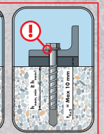
Shtrengoni bulonën e ankerimit me një çift rotullues
