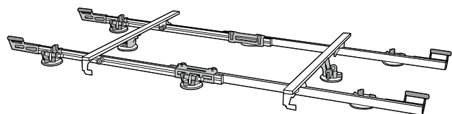
TELAIO DI MOVIMENTAZIONE DOTATO DI VENTOSE Handling frame equipped with suction cups Châssis doté de ventouses Transportrahmen mit Saugnäpfen
