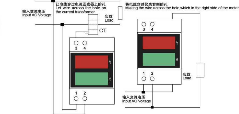
图 1: 安装电流互感器 Graph 1: install current transformer
