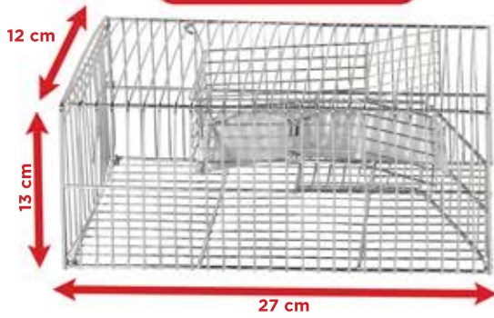
E-09 Ratoeira Pequena
