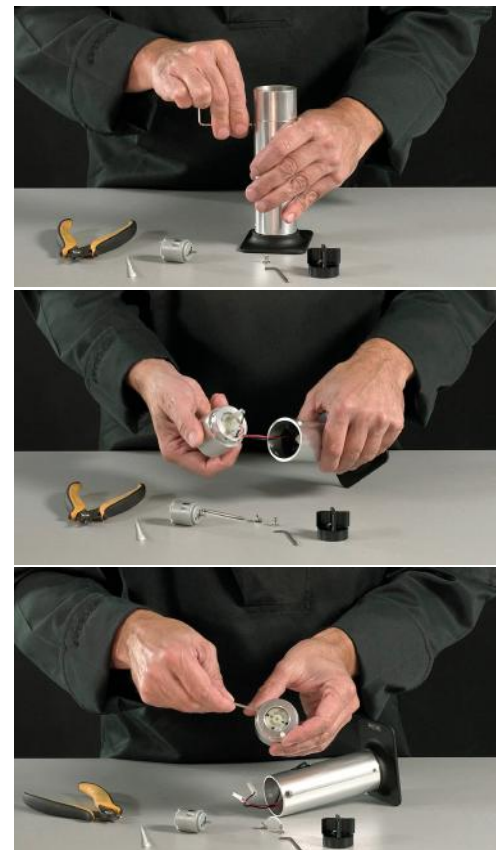
10/0048 Super Aladin & 007 Conexiones eléctricas interruptor frontal Electrical spare parts - frontal switch
