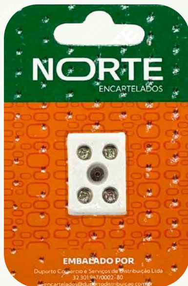
CONECTOR P/ CHUVEIRO BIPOLAR 10 mm COD: 271059
