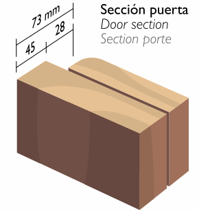
Sección puerta Door section Section porte Tabla de 28 mm. Grueso total de la hoja: 73 mm Panel thickness: 28 mm. Total door thickness: 73 mm Épaisseur du panneau: 28 mm. Épaisseur totale de la porte: 73 mm
