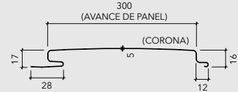
SECCIÓN PANEL 300 FS COMPUESTO
