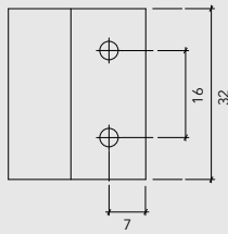
CLIP DE FIJACIÓN - PANEL 455 SL MATERIAL: ALUZINC
