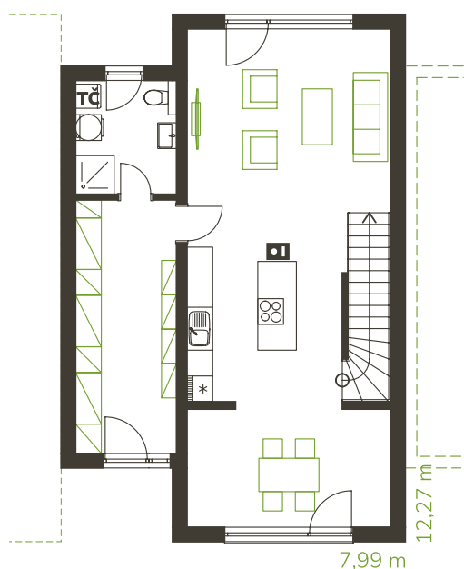
PŘÍZEMÍ
