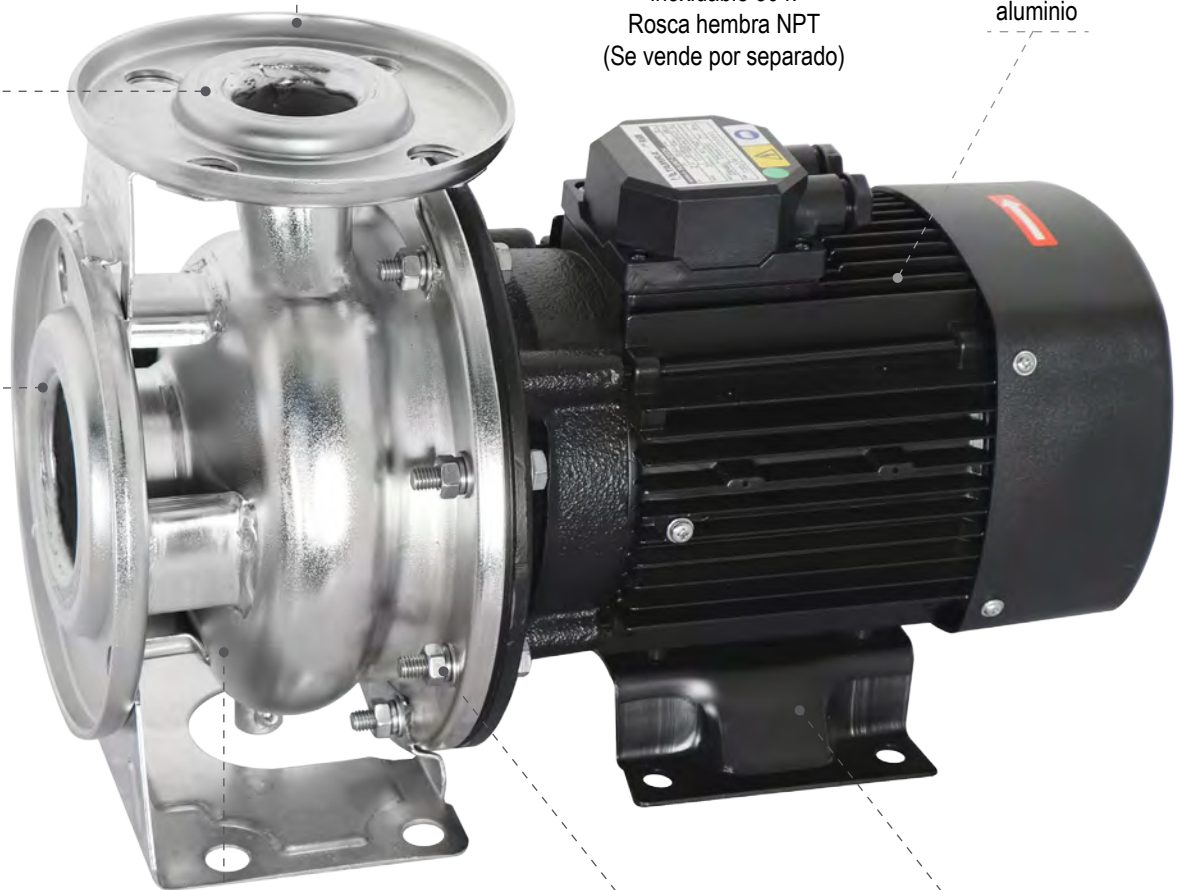
Cuerpo hidráulico en acero inoxidable 304, ideal para aplicaciones donde se requiere que el agua no tenga contacto con materiales sujetos a oxidación
