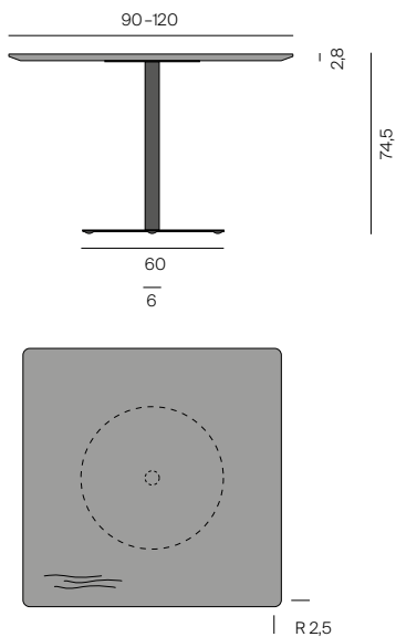
B14 quadratisch B14 square
