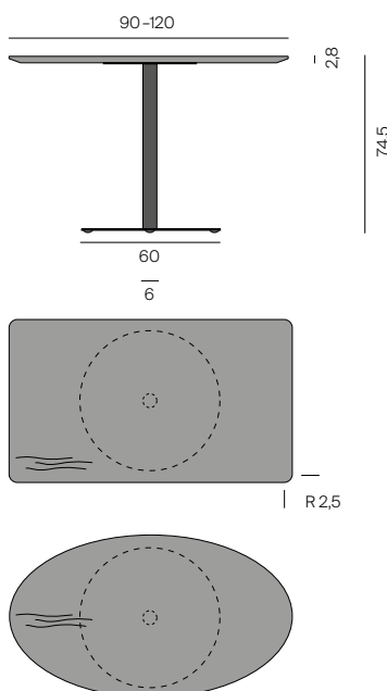
B14 rechteckig / oval, Maserung längslaufend B14 rectangular / oval, grain lengthwise
