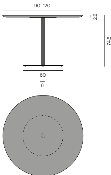
B14 rund B14 round
