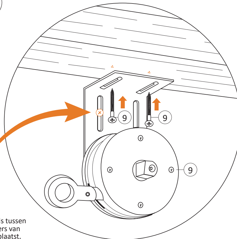
Plafondmontage
