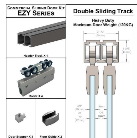
EZYS1HDD (Heavy Duty) Double Sliding Door Kit
