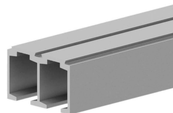
EZYS1HDD Double Sliding Door Track (118" Length)
