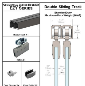
EZYS1DD Double Sliding Door Kit
