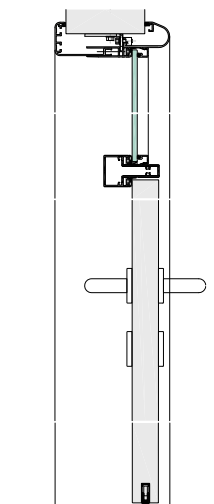
Schnitt P-P
