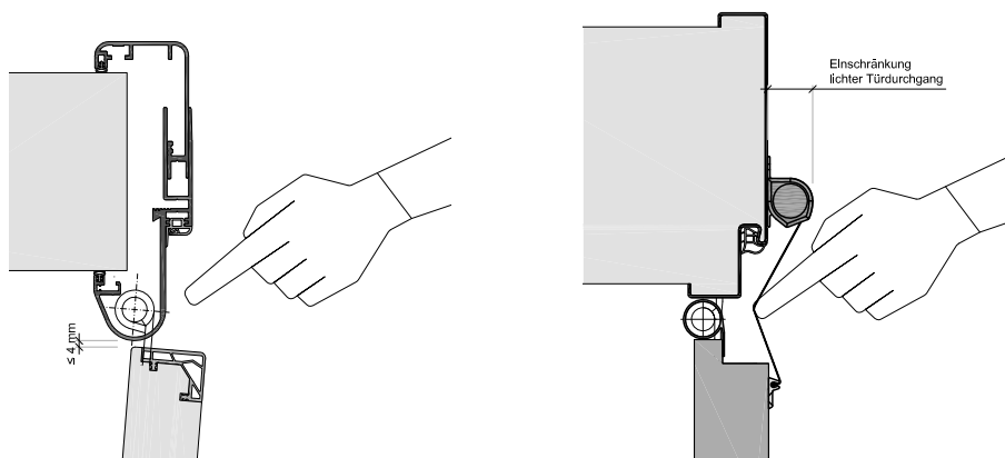
Vergleich der Nebenschließkante (Bandkante) einer Fingerschutztür mit einer Standardtür mit nachträglich aufgeschraubtem Fingerschutzrollo (Türkante gefälzt mit Überschlag) und durchgehenden Profilen zwischen den Türbändern.
