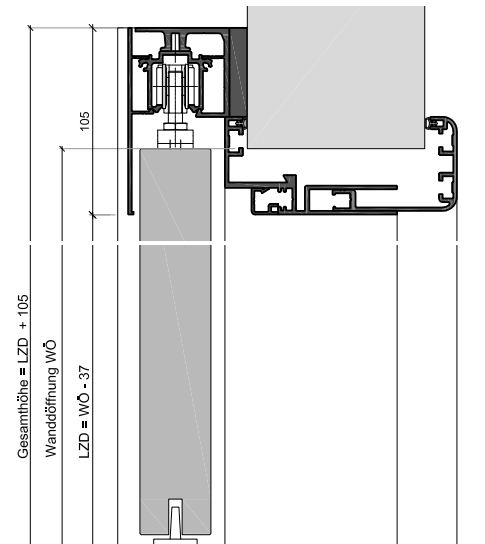
Vertikalschnitt EURORSV-42S
