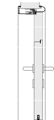
Schnitt O-O
