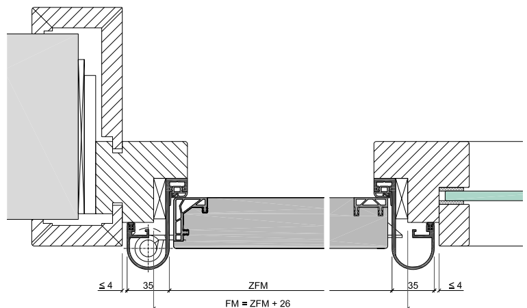
HFI Profilzarge in Verbindung mit Holzstockzarge und Verkleidungen
