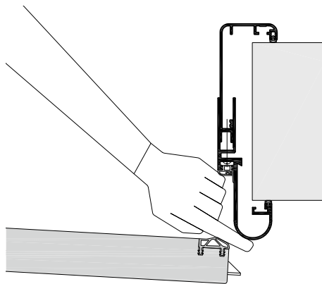
Küffner Fingerschutztür mit abgerundeter Zarge sowie integrierter Knautschzone an der Schloßkante.
