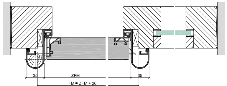
Profilzarge HFI in Holzstock- oder Blockzarge und angrenzender Verglasung
