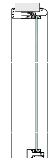
Schnitt K-K
