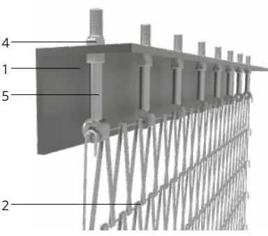
DETALLE B: FIJACIÓN INTERMEDIA
