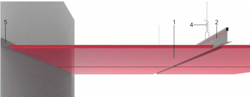
DETALLE CONTRA MURO, BANDEJA Y PERFIL AL MISMO NIVEL Y PERFILERÍA GRID ENTRE BANDEJAS
