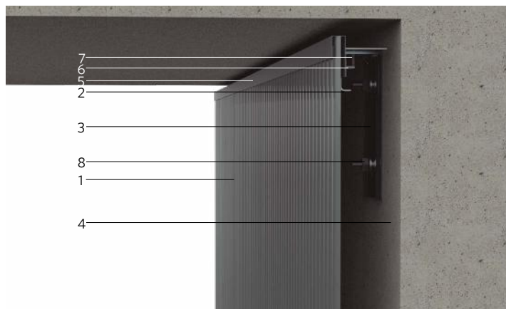
DETALLE SUPERIOR
