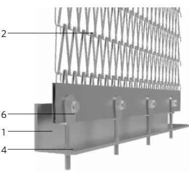
DETALLE C: FIJACIÓN INFERIOR
