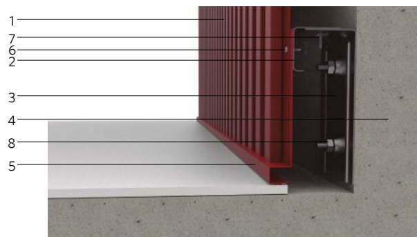
DETALLE INFERIOR
