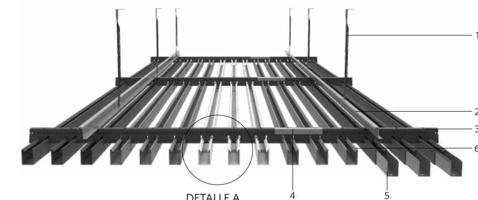
DETALLE A
