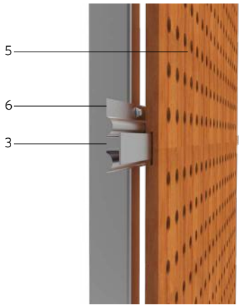
DETALLE 2
