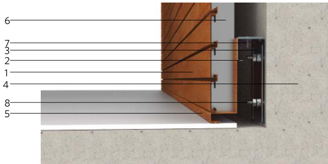
DETALLE INFERIOR
