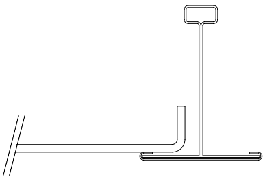
PERFIL 15/16
