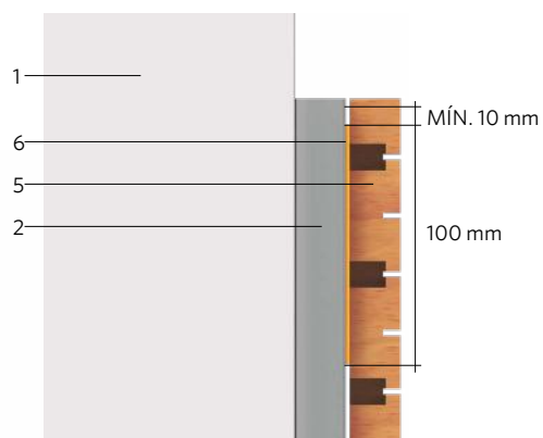
DETALLE A
