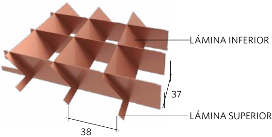
DETALLE LÁMINAS
