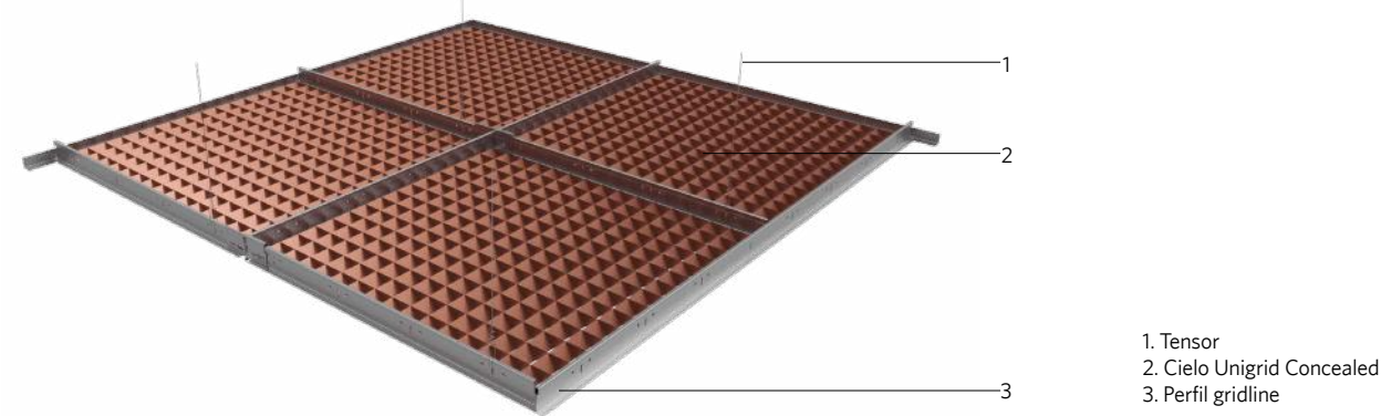
DETALLE PERSPECTIVA
