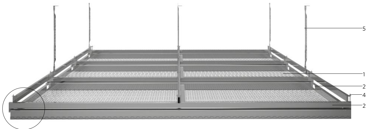
DETALLE A
