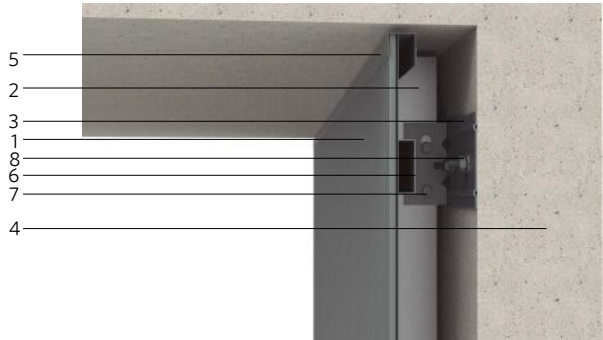
DETALLE SUPERIOR
