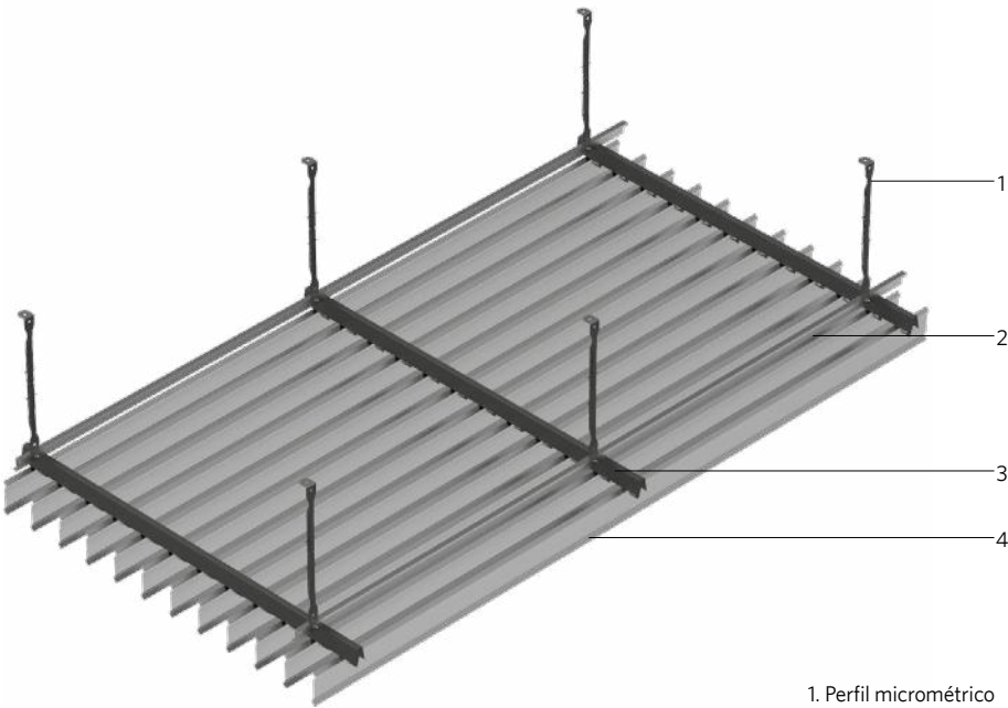
ISOMÉTRICA DE SISTEMA
