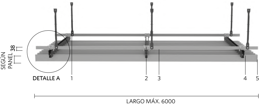
CORTE LONGITUDINAL A PANELES
