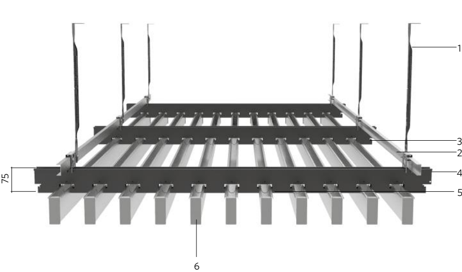
CORTE TRANSVERSAL A PANELES
