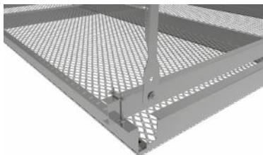
DETALLE A: PERNO U HOOK-ON
