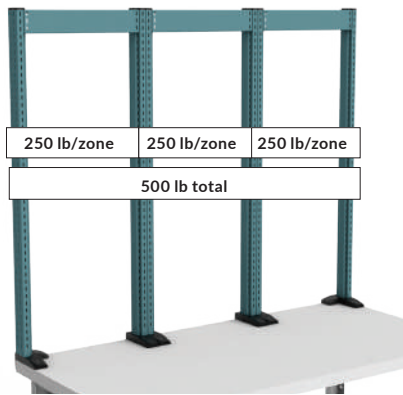
Triple frame (EW13)
