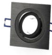
Pierścień ozdobny / Downlight ring OH28 Kobi mat czarny / matt black | IP20 | wymiary / size: 9,2 x 9,2 x 2,5 cm 002074 | EAN: 5900605097809
