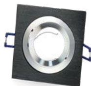
Pierścień ozdobny / Downlight ring OH28 Kobi czarny / black | IP20 | wymiary / size: 9,2 x 9,2 x 2,5 cm 002072 | EAN: 5900605093580
