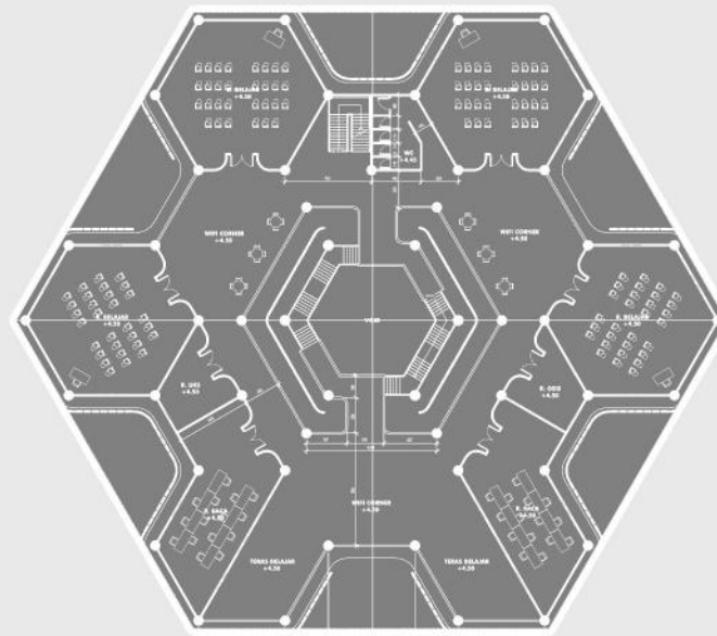
LANTAI 2
