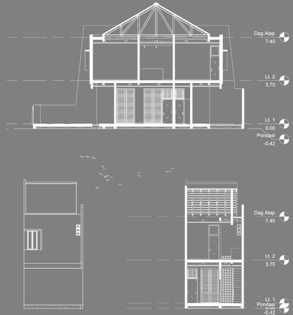
TAMPAK BELAKANG
