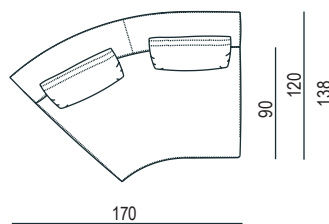
ELEMENTO SEMICURVO CON ESTENSIÓN SEMI ROUND ELEMENT WITH EXTENSION 170 X 138
