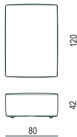
POUF OTTOMAN 80 X 120
