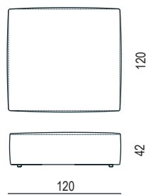
POUF OTTOMAN 120 X 120
