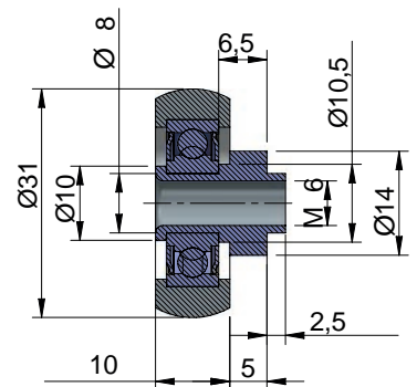
CORTE A-A
