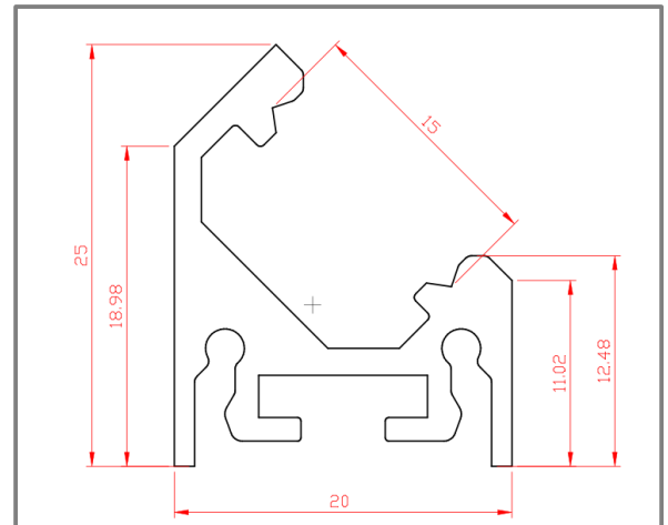
Dimensioni – Dimension H16 x L20mm
