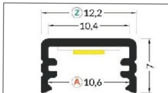
Dimensioni – Dimension H7 x L12,2 mm
