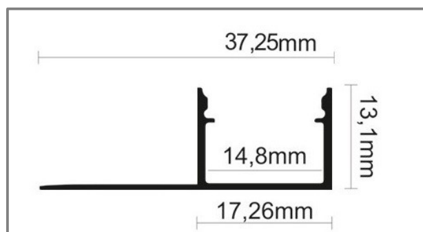
Dimensioni – Dimension H13,1 x L37,25 mm
