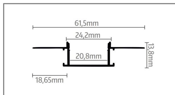
Dimensioni – Dimension H13,8 x L61,5 mm
