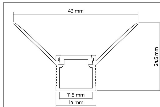
Dimensioni – Dimension H24,5 x L43 mm
