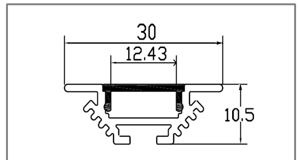
Dimensioni – Dimension H10 x L30mm
