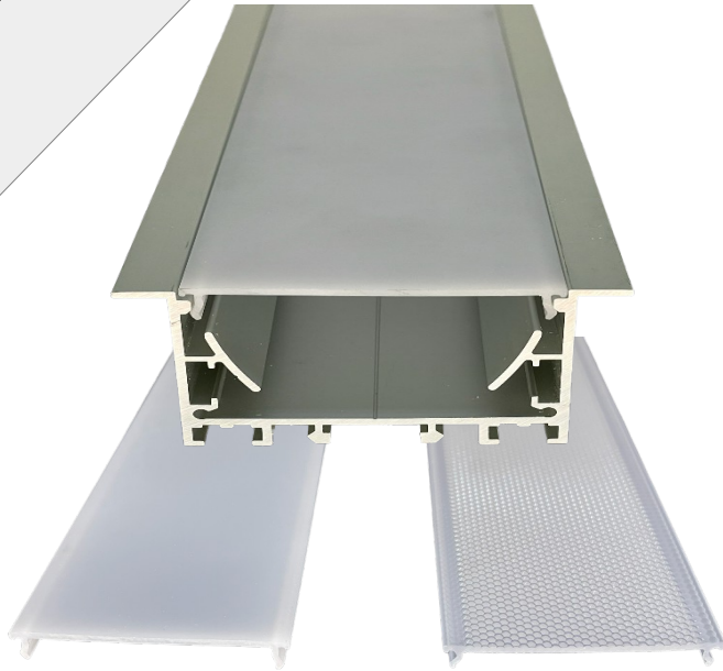
Dimensioni – Dimension H35 x L97mm
