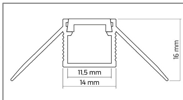
Dimensioni – Dimension H14 x L56 mm
