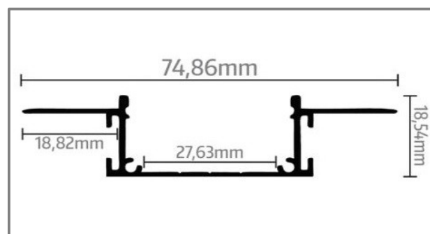
Dimensioni – Dimension H18,5 x L74,9 mm
