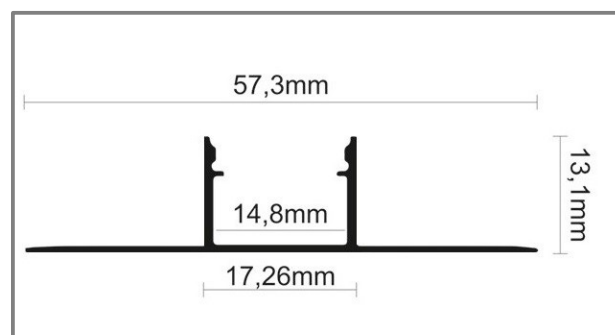
Dimensioni – Dimension H113,1 x L57,3mm
