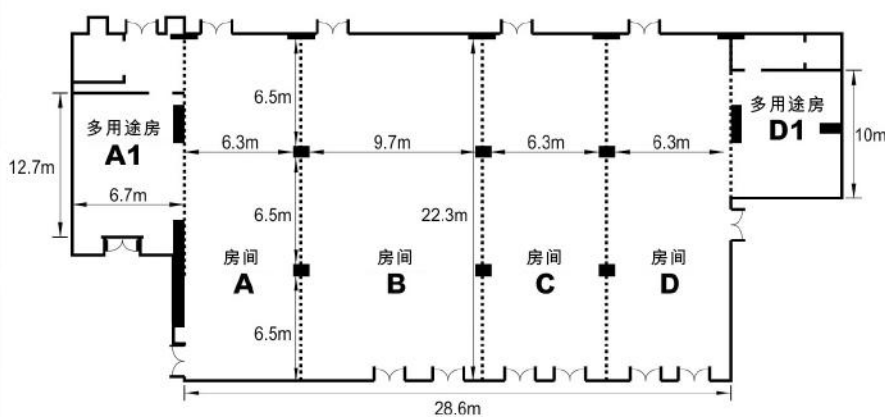
宴会厅 - 平面图(700平方米)
