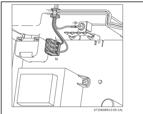
Fig. 33 Conexiones del cable de alimentación
