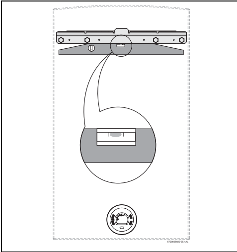
Fig. 18 Fijar la barra de fijación
