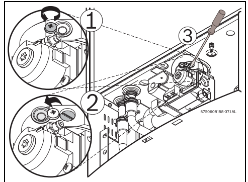
Fig. 40 Ajuste de CO 2 en modo P1
