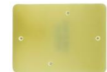
pbs42510 Produktschutzplatte SP 190 / Isolation plate SP 190 173 x 127 x 5 mm 4 Senkbohrungen / 4 countersunk holes
