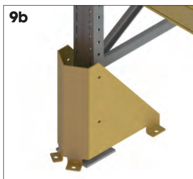
9b Staanderbescherming om de stelling geplaatst.
