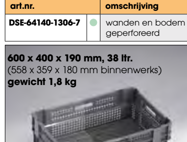
600 x 400 x 190 mm, 38 ltr. (558 x 359 x 180 mm binnenwerks) gewicht 1,8 kg
