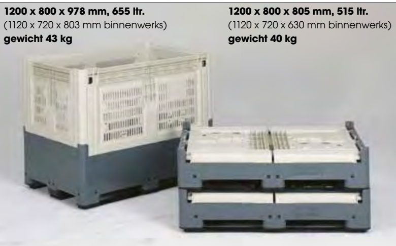
Europallet compatibele Smartboxen.
