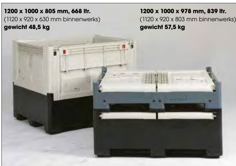
Blokpallet compatibele Smartboxen.
