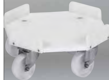
transportroller, achthoekig uit 15 m dik PE met 4 opstaande randen van 70 mm
