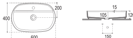
ORBIT 60 x 40 εκ. 31060-300 205,00€ Αποστάτης (για μπαταρία με A/B) SPAC/L2 25,00€
