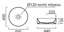
Χωρίς υπερχειλίση Βάθος γούρνας: 11εκ.
