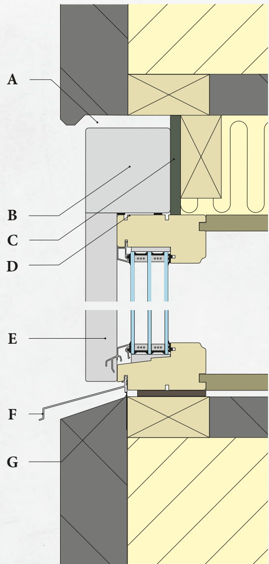
NorDan Screens montert i murfasade
