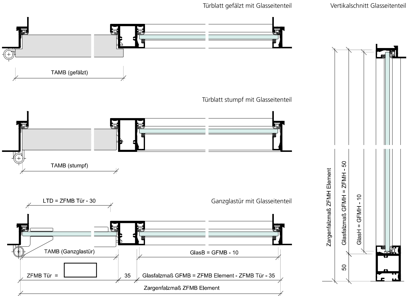
Türblätter, Beschläge und Glas nicht im Lieferumfang. Darstellung: DIN Links (DIN Rechts spiegelbildlich)
