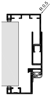
Umfassungszarge EUROKF / EUROKS (gefälzt / stumpf)
