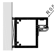
Blockzarge BF / BS (gefälzt / stumpf)
