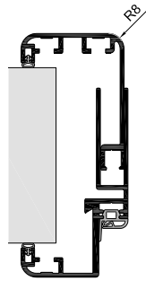
Umfassungszarge EURORF / EURORS (gefälzt / stumpf)
