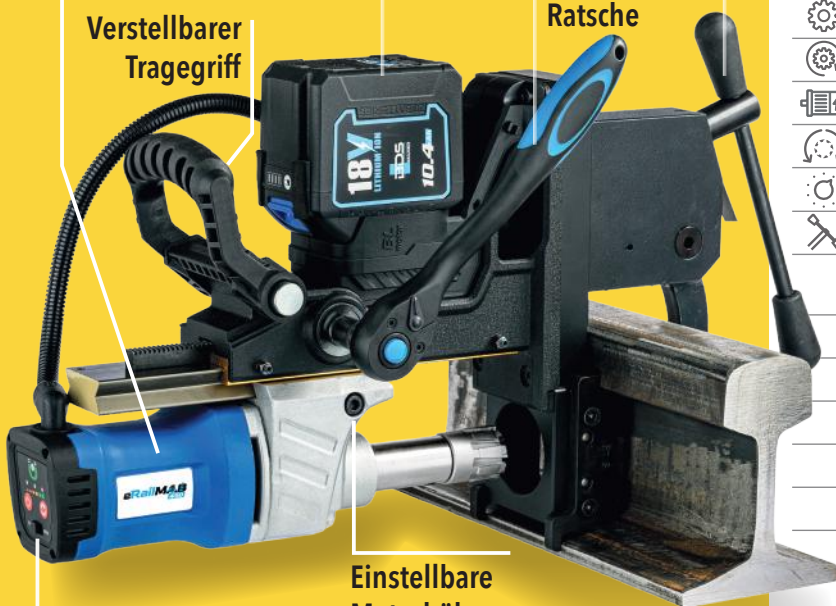
Bürstenloser Motor
