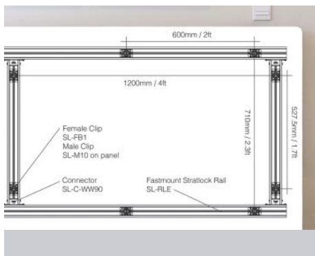
Solution de montage de panneaux : SL-FB1 & SL-RLE - structure & SL-M10 - panneau
