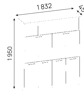
ТУМБА СЕРВИСНАЯ
