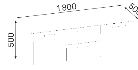
ТУМБА СЕРВИСНАЯ
