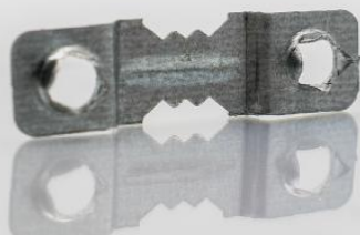
K7 - Zawieszka wciskana na dwie rozety 12x41mm
