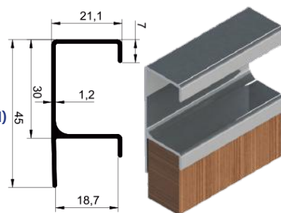
PUXADOR PERFIL ALUMÍNIO DES-960 G-18 PARA 18MM (UN) 3203 ANODIZADO 6MT
