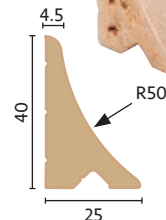
QW-RD40 Door Rain Deflector
