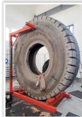
▲ R49-R57 хэмжээтэй дугуй засварын моторт ажлын тавцан
