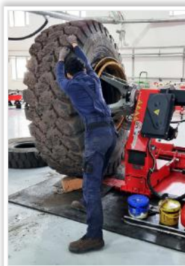
▲ R35 хүртэлх хэмжээтэй дугуйг задлаж, угсрах алсын удирдлагатай бүрэн автомат PROMAXX машин
