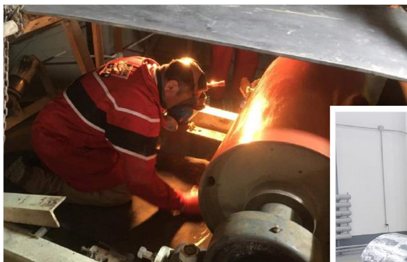
1600 мм өргөнтэй, 630мм голчтой хөтлөгч булыг 12 мм зузаантай REMAGRIP 60/CN резинээр хуяглахад бэлтгэн металл гадаргуун цэвэрлэгээг хийж буй байдал
