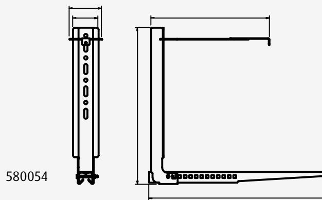
Säädettävä kannake
