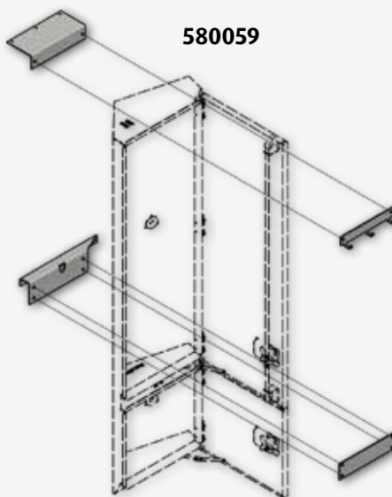
KANNATIN RST BevoBox™ Vasen Scania
