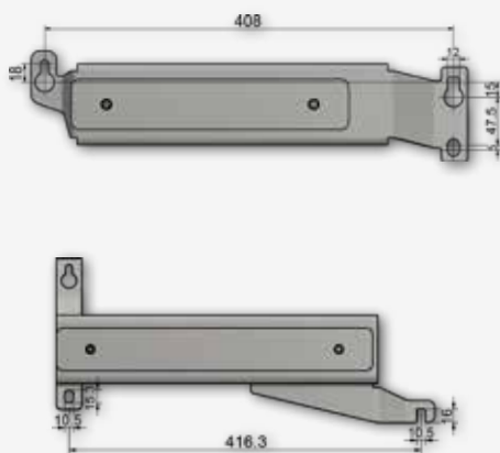
KANNATIN Galvanoitu BevoBox™ Oikea Scania
