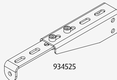
Lisätuki
