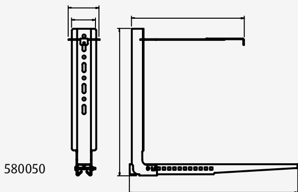
Säädettävä kannake
