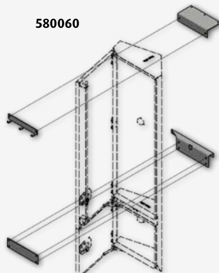
KANNATIN RST BevoBox™ Oikea Scania
