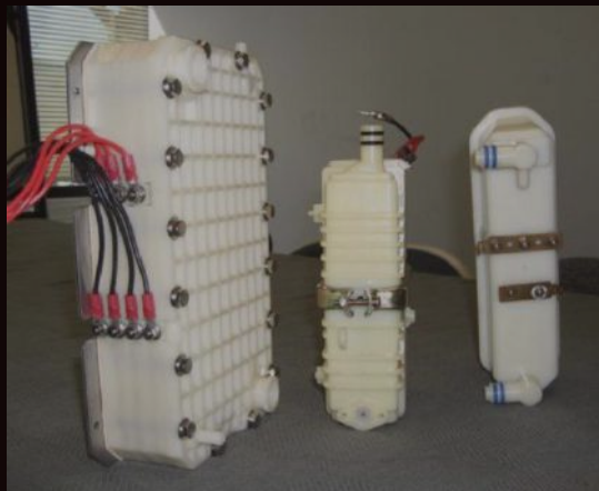
Chambres d'électrolyse : Kangen (grande, gauche) vs copies (petites, droite)
