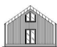
ELEWACJA SZCZYTOWA
