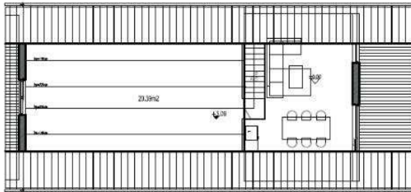
RZUT ANTRESOLI
