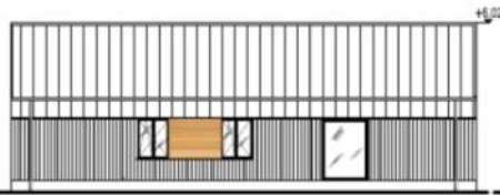
ELEWACJA OGRODOWA
