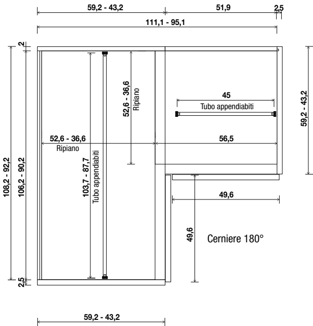
Elemento angolo anta da 49,6 cm
