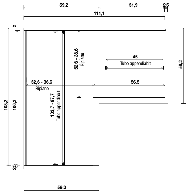
Elemento angolo 49,6 x 49,6 cm solo per Cabina Telaio
