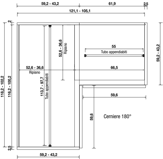
Elemento angolo anta da 59,6 cm
