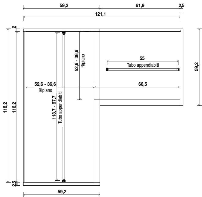
Elemento angolo 59,6 x 59,6 cm solo per Cabina Telaio
