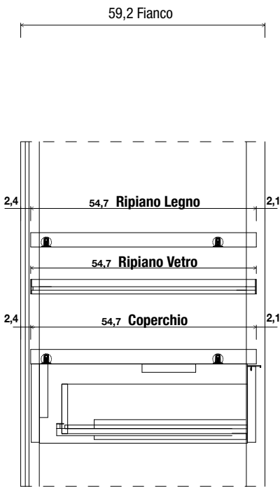
Per ante battenti schienale vetro
