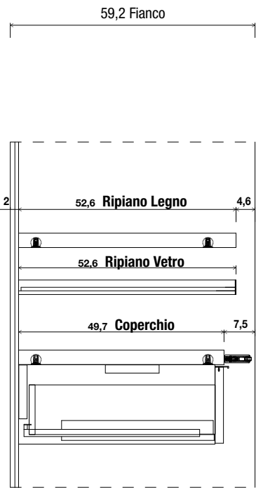
Per ante battenti legno
