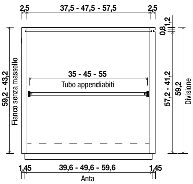
Elemento anta singola
