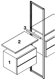
Accostamento fianco/divisione Telaio
