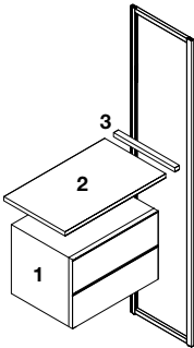
Accostamento fianco/divisione Telaio
