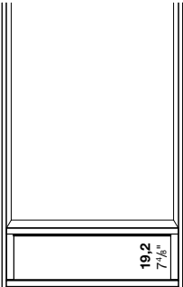
1 cassetto a terra
