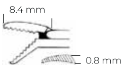
RICHARDS MCK 06.105.35 left tip / sol uçlu straight shaft / düz şaft 8 cm
